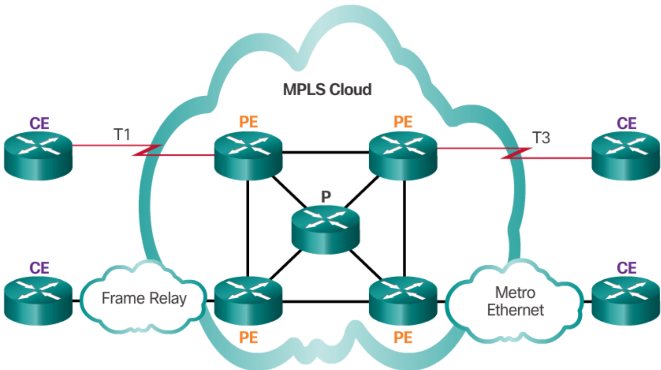
სურ. 4.3.1 - მარტივი MPLS ტოპოლოგია
