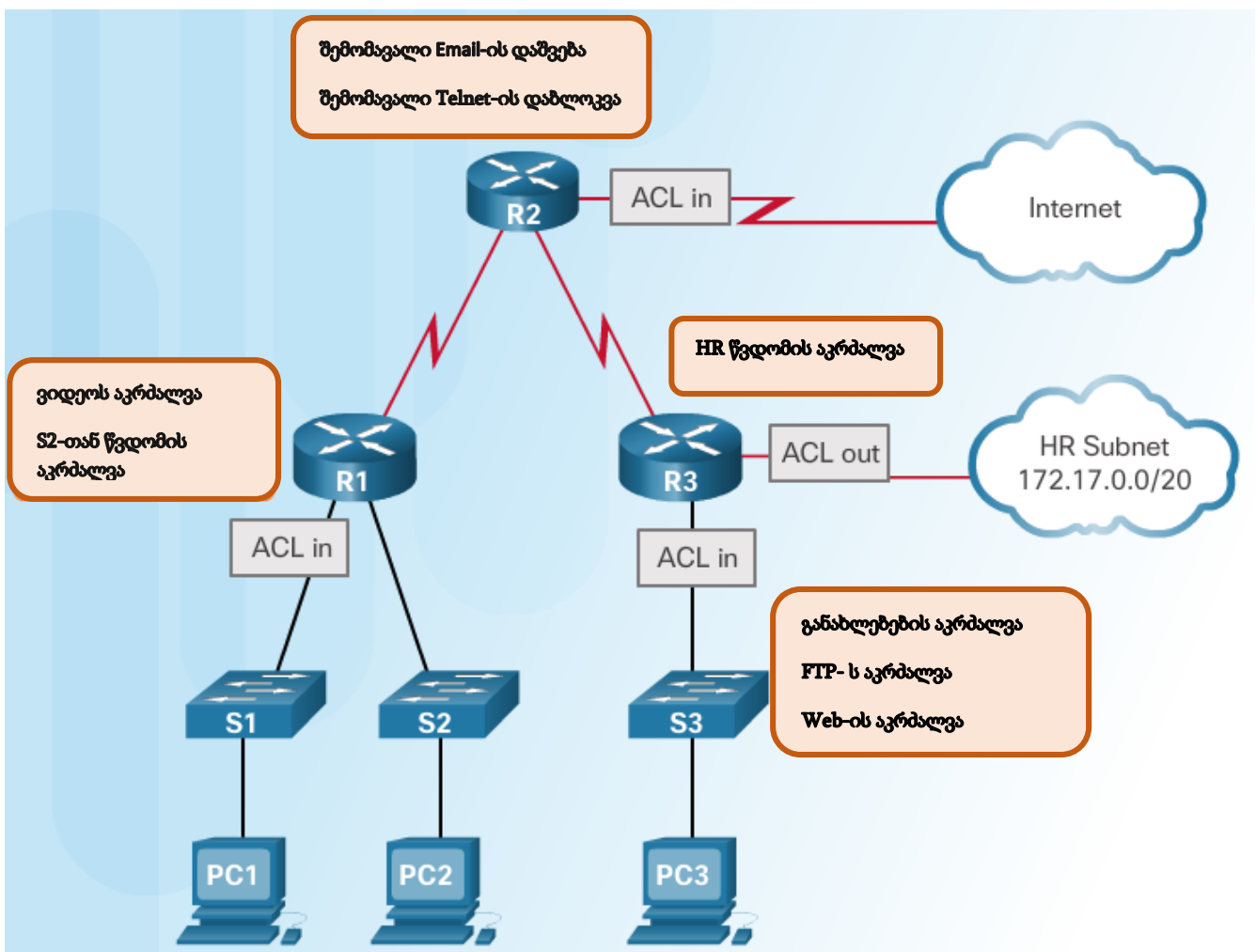
სურ. 3.2.1. წვდომის კონტროლის სია (ACL)
