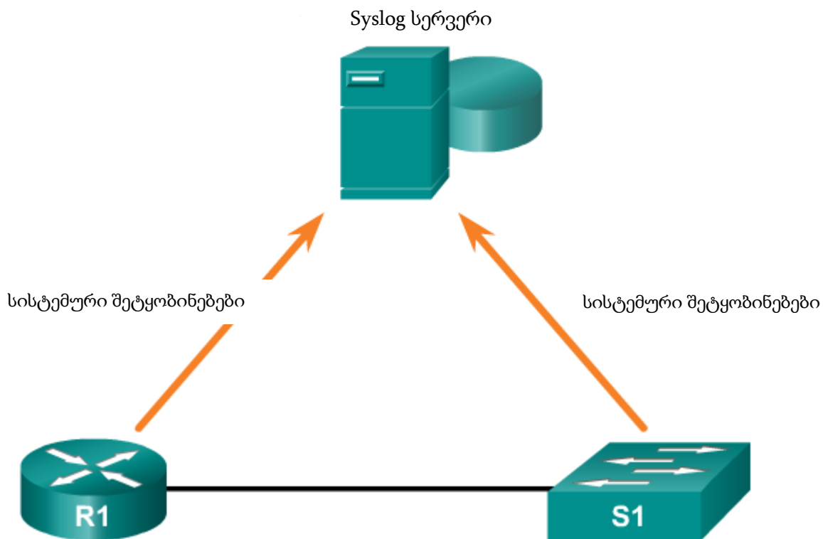
სურ. 6.3.2.1 Syslog
